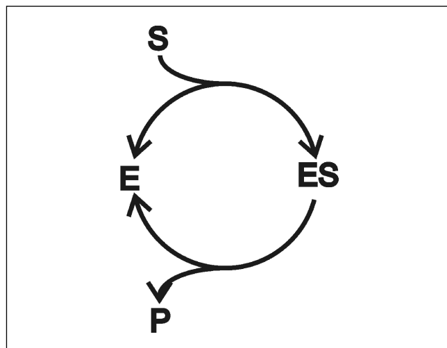
Figura 8. Representación esquemática de un ciclo de catálisis.
